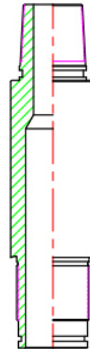
BOTTOM SUB PART #: FJ-3625BB-04
